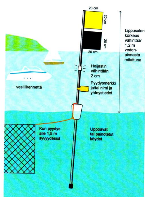
Kuva 2. Pintapyydys eli lähemmäksi kuin 1,5 metriä veden pintaa ulottuva pyydys, tulee vesiliikenteen käyttämissä alueilla merkittä kahdella päällekkäin kiinnitetyllä lipulla. (Piiros Anu Väitalo/KKL)
