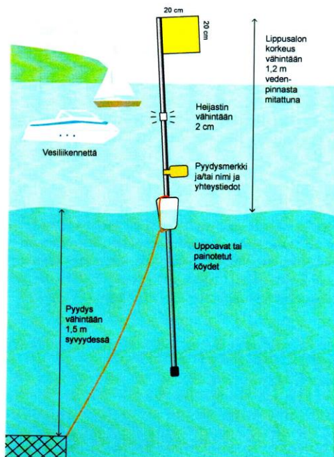
Kuva 1. Vesiliikenteen käyttämissä alueilla pyydys on merkittävä 1,2 metriä vedenpinnan yläpuolelle ulottuva salkoon kiinnitetyllä vähintään 20 senttimetriä leveällä ja korkealla neliön muotoisella lipulla. (Piiros Anu Väitalo/KKL)
